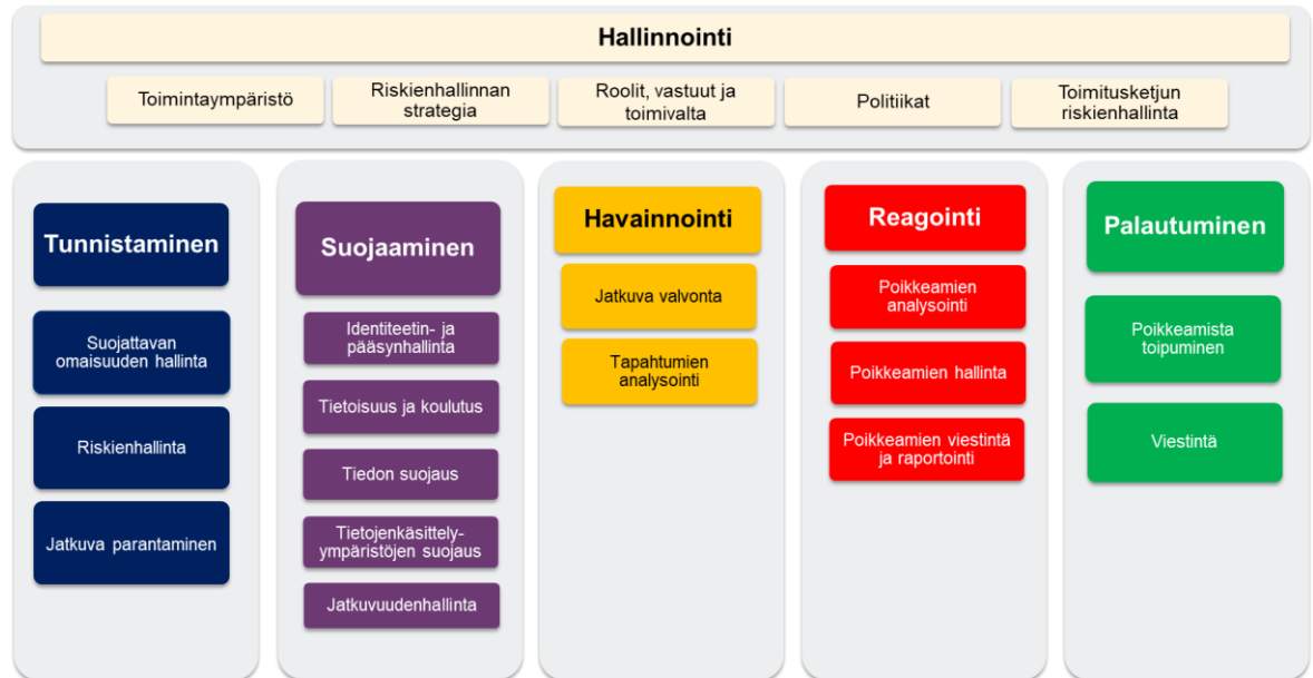
Kuva 3 Digitaalisen turvallisuuden arkkitehtuurin viitekehys
